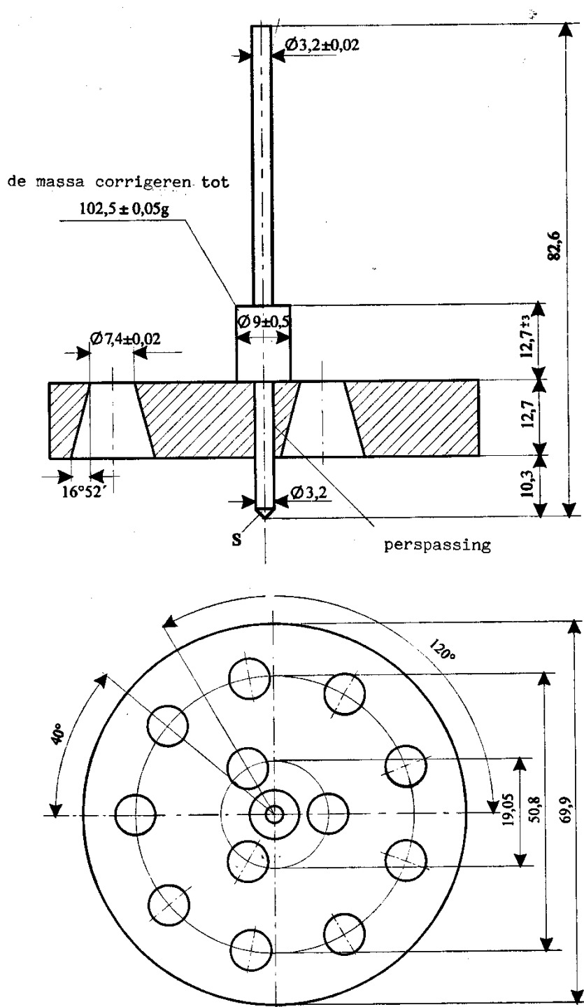
Figuur 1 Penetrometer
